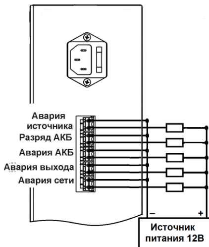
Рисунок 2 – Подключение внешних устройств автоматики
