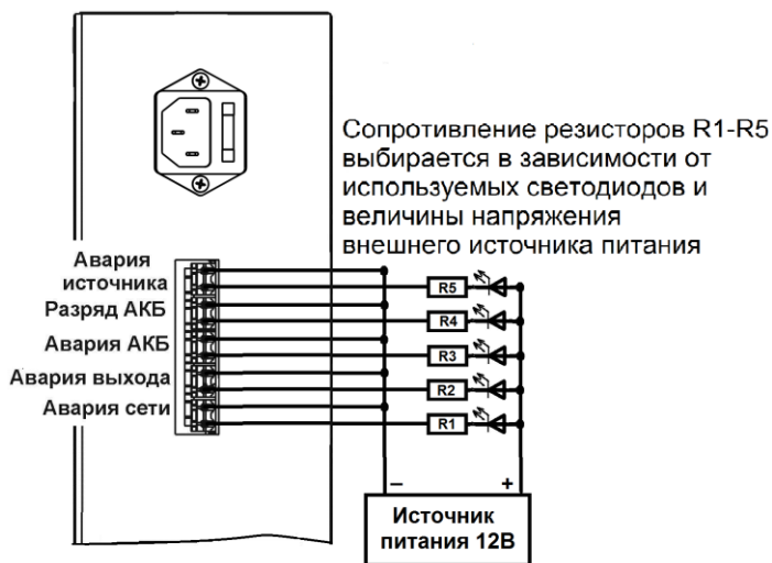
Рисунок 2 – Подключение внешних устройств автоматики
